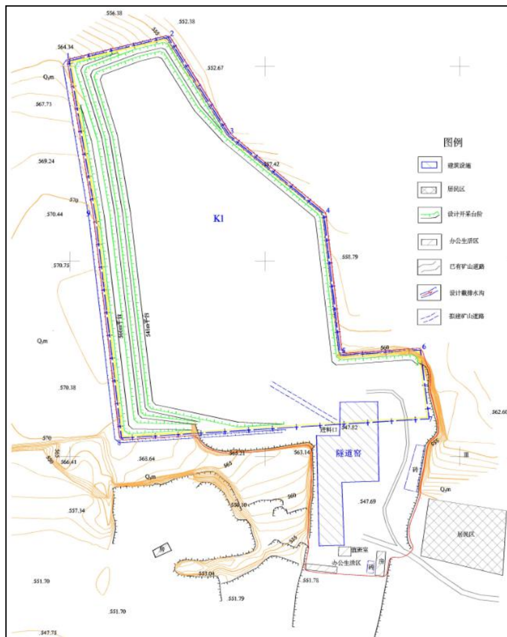
矿山工程平面布置示意图
