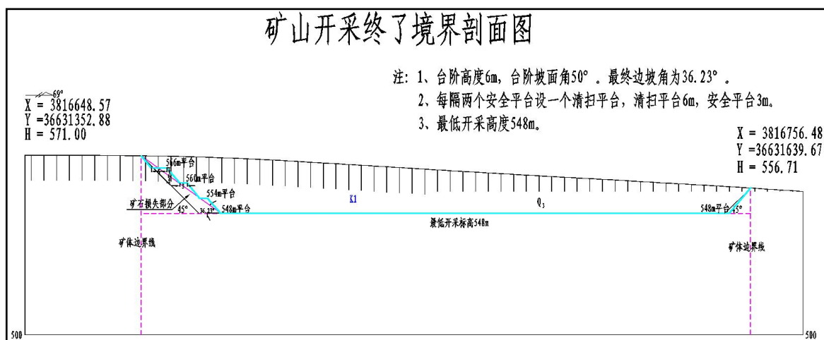
图 1.3-2 开采终了剖面图
